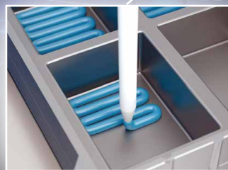
バッテリーケースに2液性ギャップフィラーを塗布
